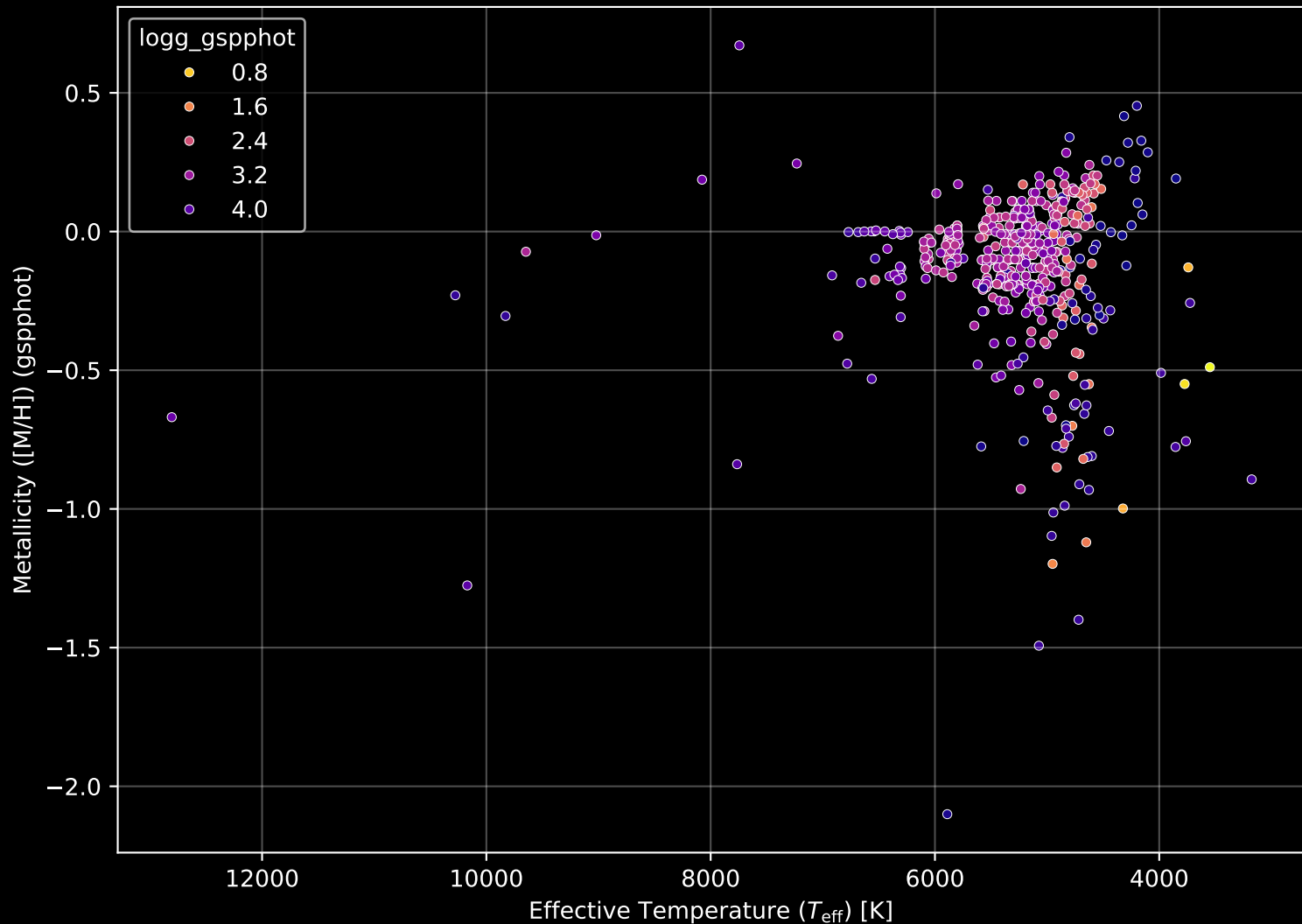
APOGEE DR17 Field: [180-08] Stellar Population Parameters (n= 503)
